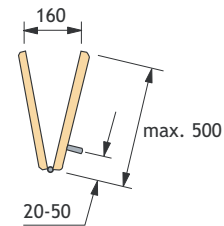
Vouwdeur 2 vleugels
