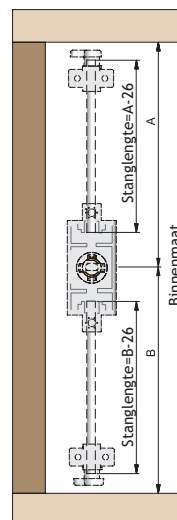
Uitsparingsafmeting
