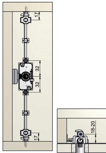
Technische tekening
