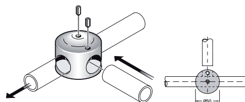
T-verbodingsstuk 3 wegbuizen.
