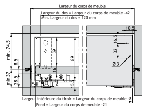
Mesures d'encastrement d'un tiroir intérieur
