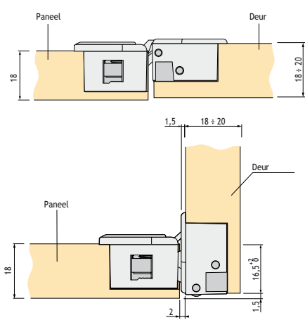
Paneeldikte 18 mm
