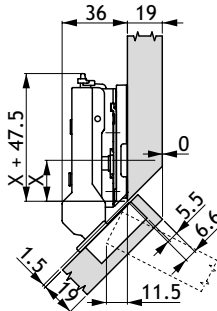
Montageplaathoogte 8
