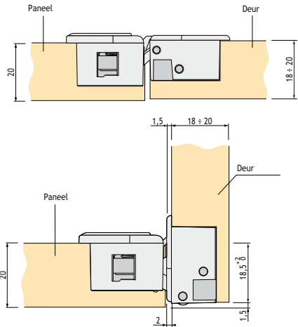
Paneeldikte 20 mm
