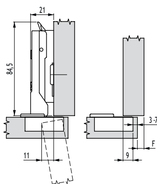
Montageplaathoogte 3
