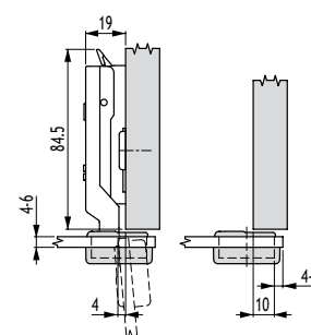
Montageplaathoogte 2
