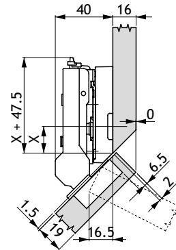
Montageplaathoogte 12
