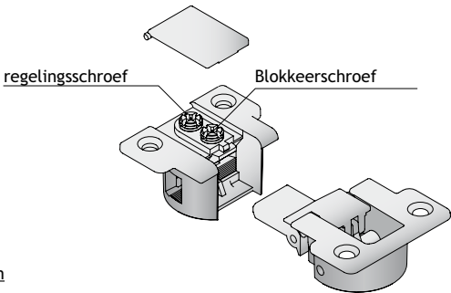
Paneeldikte 18 mm
